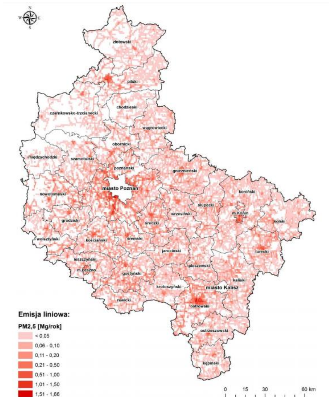
Rysunek 6 Lokalizacja i wielkość emisji pyłu PM 2,5 ze źródeł liniowych na terenie strefy wielkopolskiej;
