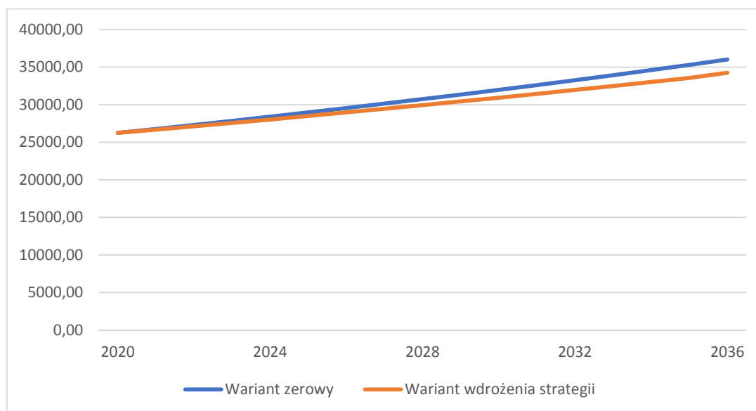
Rysunek 13 Emisja dwutlenku węgla z transportu - porównanie wariantów (dane w Mg CO 2 )
