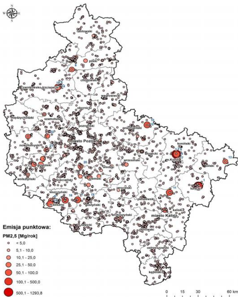
Rysunek 5 Lokalizacja i wielkość emisji pyłu PM 2,5 ze źródeł punktowych na terenie strefy wielkopolskiej; źródło: Program ochrony powietrza dla strefy wielkopolskiej w zakresie pyłu PM 10 , PM 2,5 oraz B(a)P
