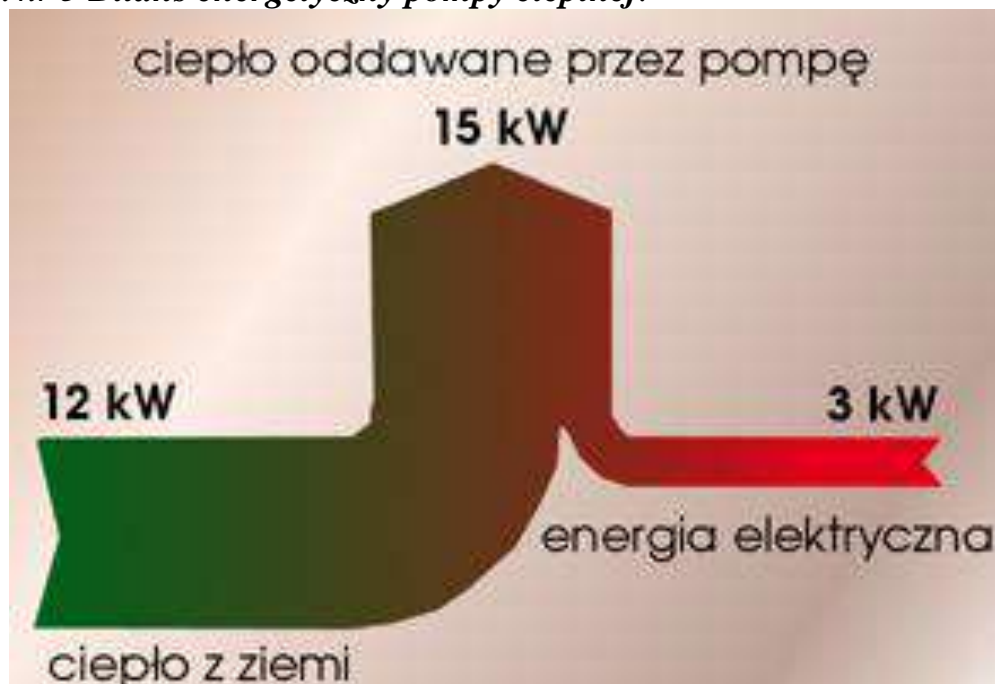
Rysunek nr 5 Bilans energetyczny pompy ciepłej:
