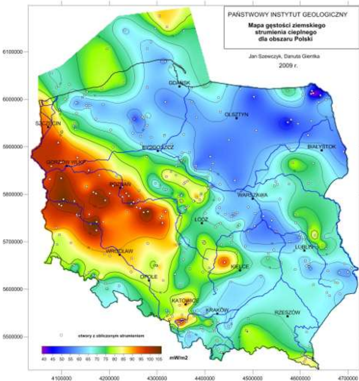
Rysunek nr 9 Mapa strumienia ciepłego dla obszaru Polski. Źródło: www.pig.gov.pl (J. Szewczyk, D. Gienka, PIG 2009)
