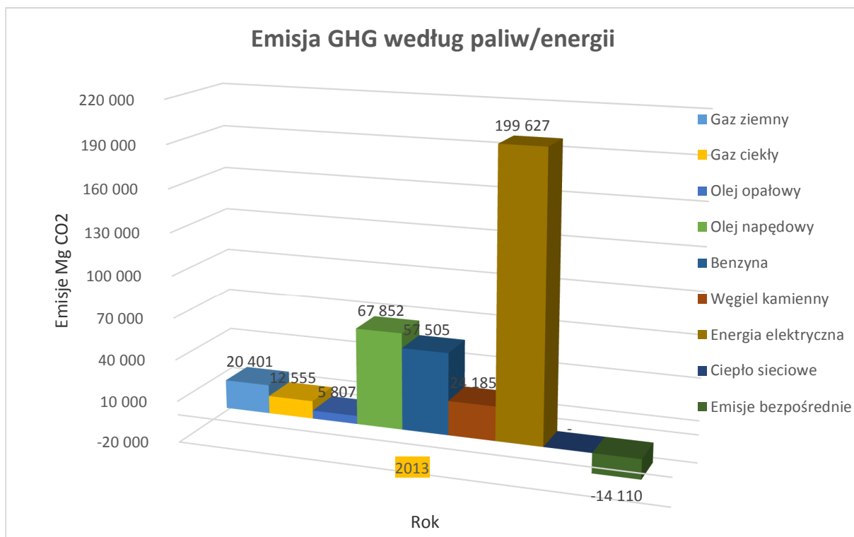
Rysunek 13 Wielkość emisji CO 2 z terenu gminy Śrem w 2013 roku wg źródeł energii
