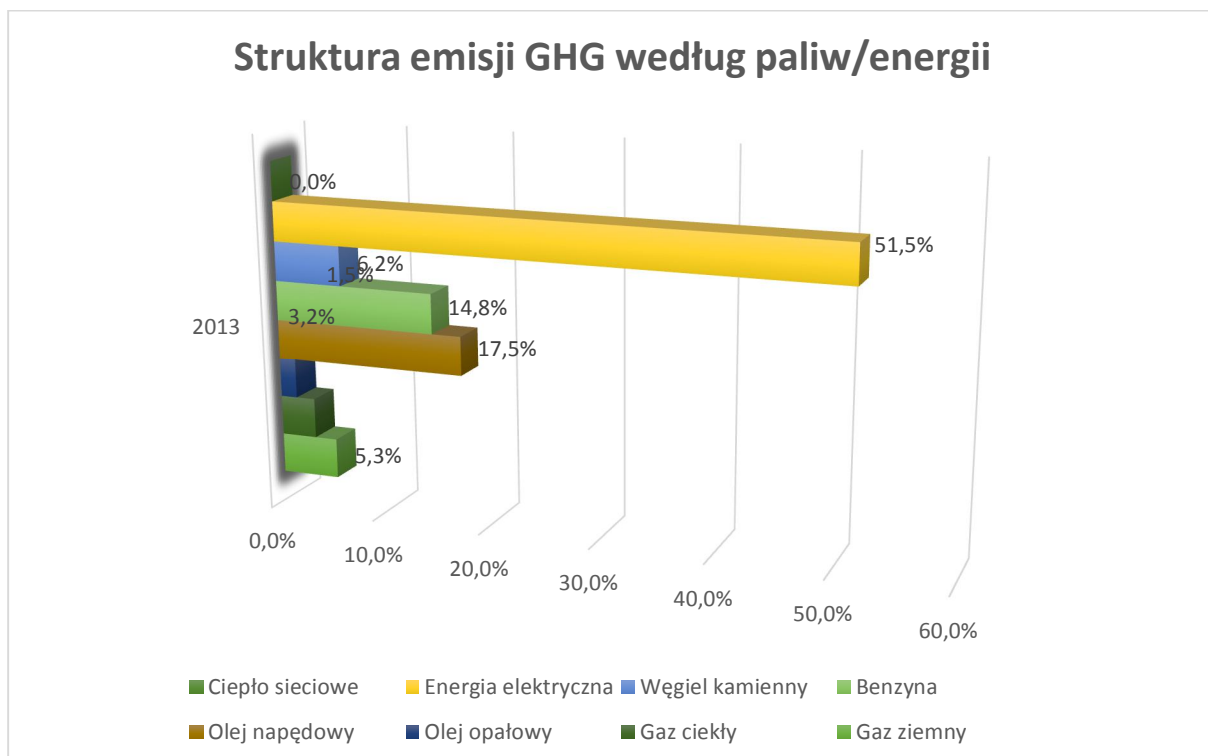
Rysunek 14 Procentowy udział źródeł energii w całkowitej emisji CO 2 z terenu gminy Śrem w 2013 roku
