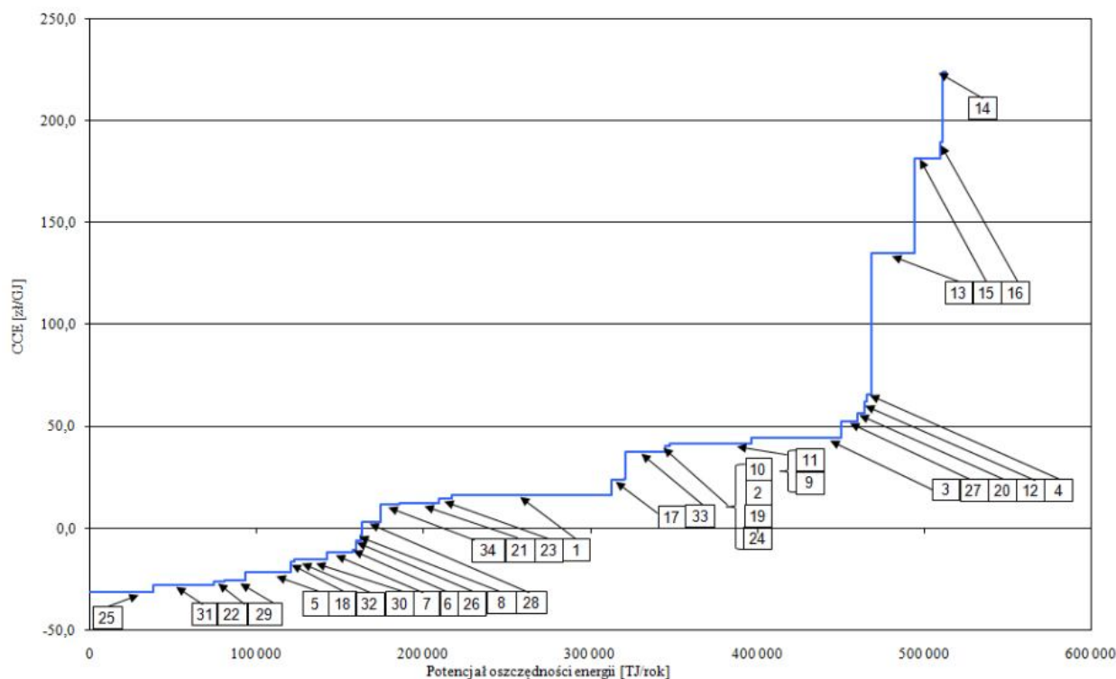
Rysunek 18. Potencjał oszczędności energii w budynkach w Polsce. Objasnienia oznaczeń w Tabela 35
