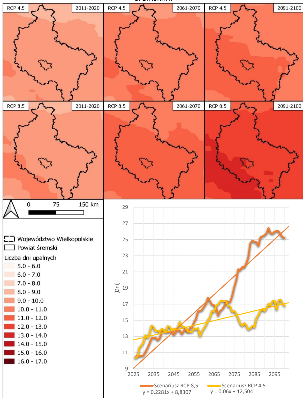
Figura 2.5. Średnia krocząca liczby dni upalnych ( T_{max} > 30^{\circ}\text{C} ) w powiecie śremskim.
